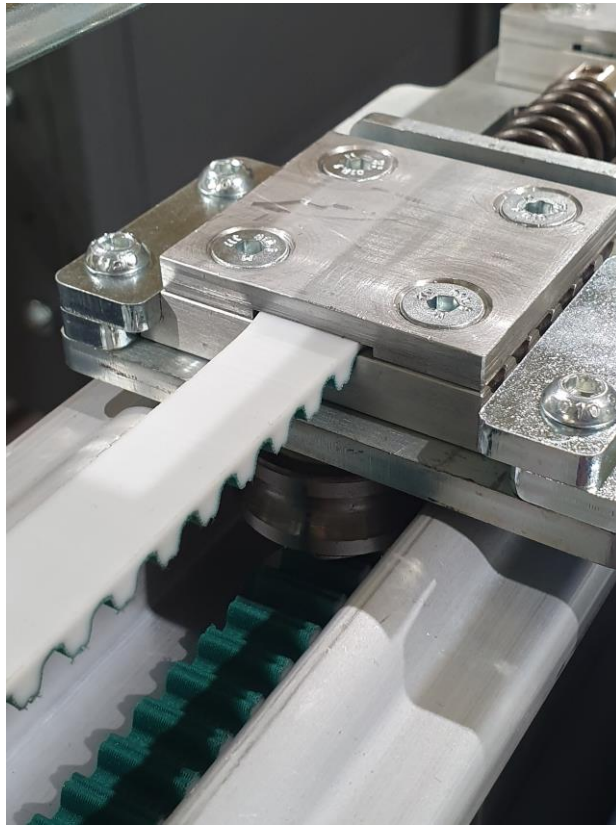
Zahnriemen von oben Timing Belt from the top
